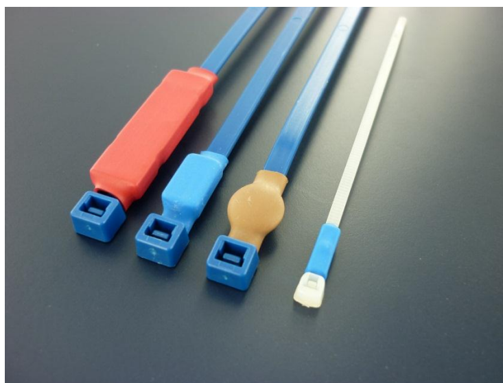
smart-DOME Classic Kabelbinderlösungen mit integrierter UHF- und HF-Technologie (2x UHF- und 2 HF-Versionen v.l.n.r.)
